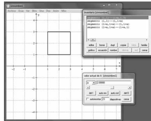
Figura 1. Construcción de un cuadrado de longitud a .
