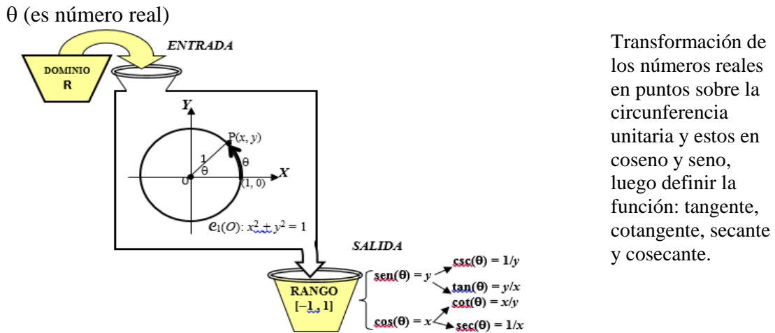
Figura 1. Máquina productora de las funciones seno y coseno de \mathbf{R} en [-1, 1]
