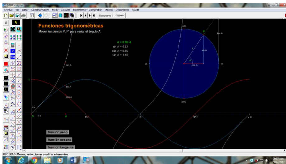
Figura 2. Gráfica de la función coseno, seno y tangente en correspondencia con puntos sobre la circunferencia unitaria.
