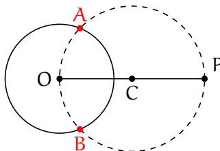
Figura 1.27: Rectas Tangentes a un círculo desde un punto exterior
