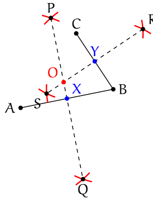
Figura 1.22: Definición del punto O
