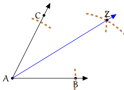
Figura 1.16: Bisección de un ángulo
