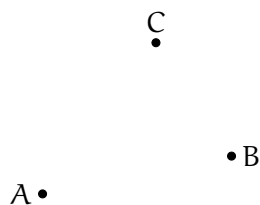
Figura 1.20: Los puntos A, B y C
