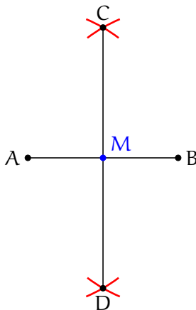
Figura 1.19: Punto Medio M
