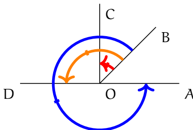
Figura 1.7: Trazado de diferentes ángulos
