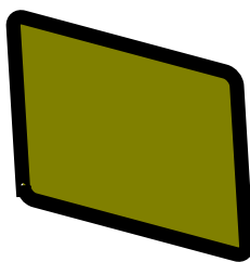
Figura 1.8: Trazado de un polígono
