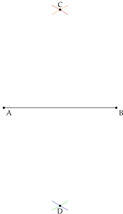
Figura 1.14: Primera Marca Triángulo Equilátero
