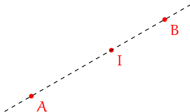
Figura 1.10: Coordenadas Baricéntricas con dos puntos
