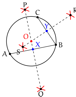
Figura 1.23: Círculo que pasa por A, B y C
