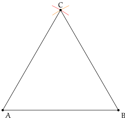
Figura 1.15: Triángulo Equilátero Listo
