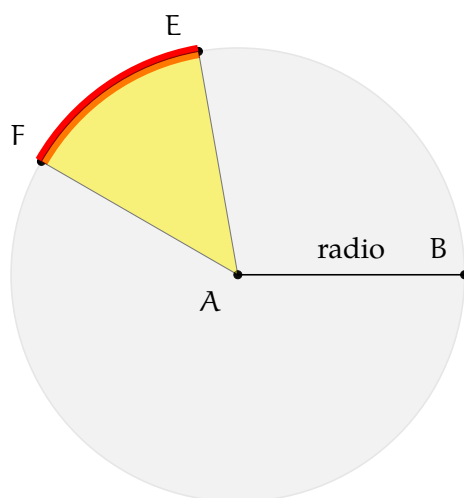
Figura 1.5: Círculo, arco y sector
