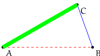
Figura 1.3: Definición de segmentos
