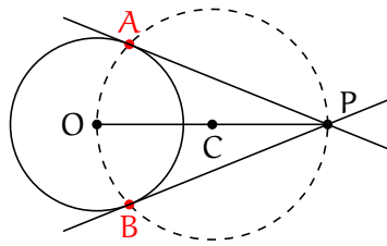
Figura 1.28: Rectas Tangentes a un círculo desde un punto exterior
