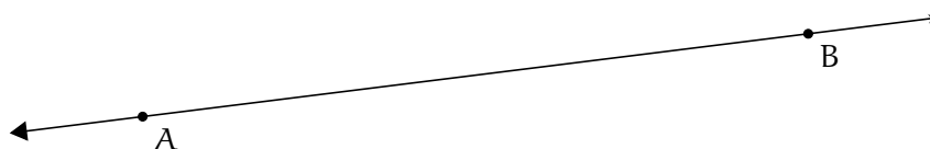
Figura 1.4: Definición de recta
