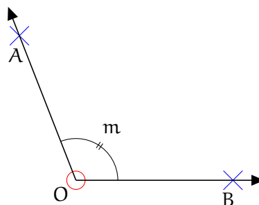
Figura 1.6: Representación de un ángulo
