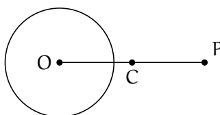
Figura 1.26: Definición del Punto medio C
