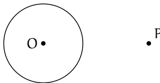
Figura 1.25: Círculo K y punto exterior P
