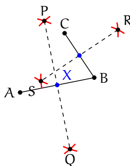
Figura 1.21: Construcción de las mediatrices
