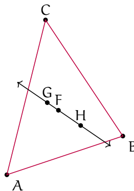
Figura 1.11: Recta de Euler
