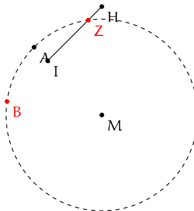
Figura 1.9: Definición extendida de puntos
