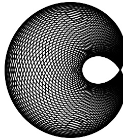
Figura 1.29: Caracol con hoyuelo
