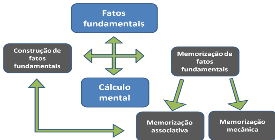
Figura 1: Relação entre fatos fundamentais e cálculo mental
