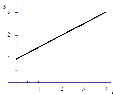
Figura 7. Primer esbozo de la Grafica de s(t) = 0.5t + 1
