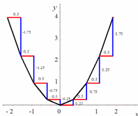
Figura 14. Representación de las diferencias, \Delta x y \Delta y , para \Delta x = 0.5
