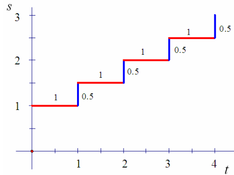
Figura 5. Representación de las diferencias: \Delta t y \Delta s , para \Delta t = 1
