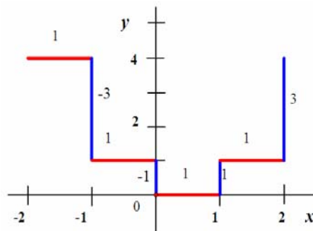
Figura 11. Para \Delta x = 1 , representación de algunas diferencias, \Delta x y \Delta y .
