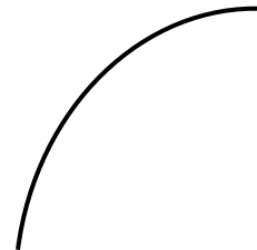
Figura 3. Curva con “lados infinitamente pequeños”
