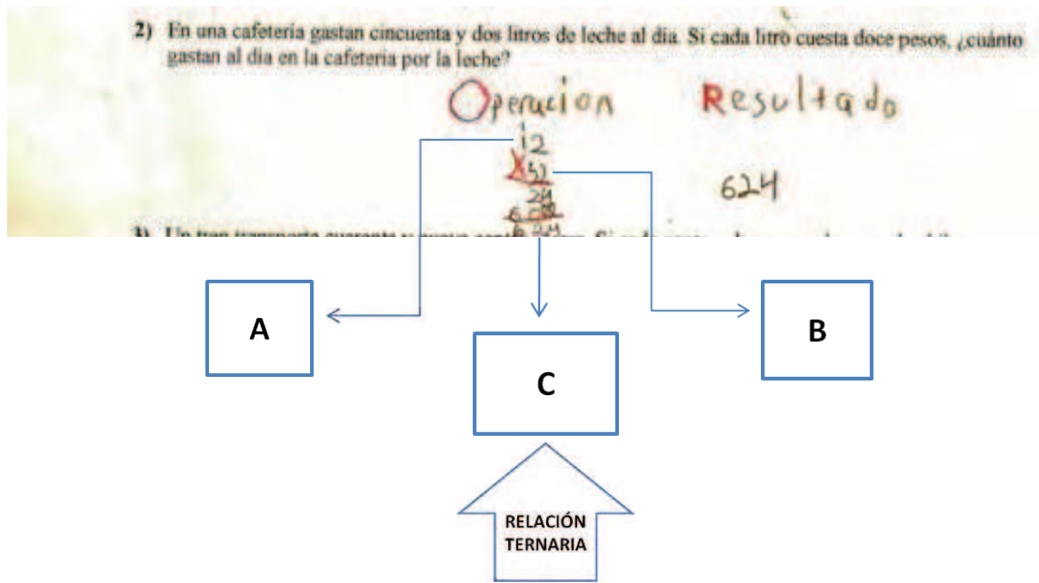
Figura 3. Relación ternaria
