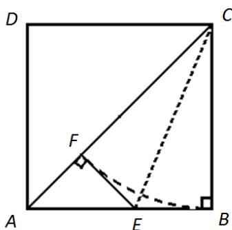
Figura 6 Cuadrado ABCD
