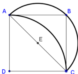
Figura 3: Cuadratura de la lúnula
