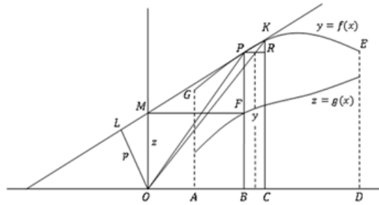
Figura 27: Método de Transmutación 23
