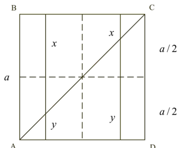
Figura 14: Medida de un cuadrado 5
