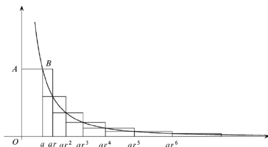
Figura 15: Cuadratura de la Hipérbola por Fermat
