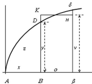
Figura 19: Cuadratura de la curva AD\delta 12
