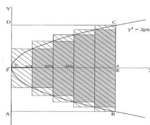
Figura 42: Volumen del paraboloides de revolución
