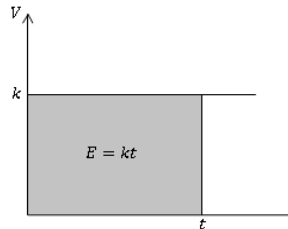
Figura 20: Área desde la perspectiva de Newton 14
