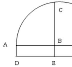
Figura 23: Fluxiones y fuentes 17
