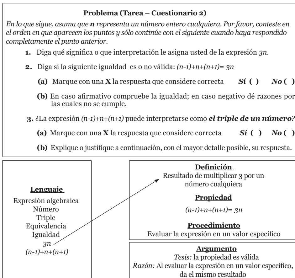
Diagrama 5.13. Configuración inicial de Cristian: E_1^{9,1}
