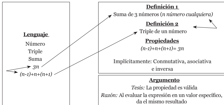
Diagrama 5.15. Configuración inicial de Dairon: E_3^{9.1}
