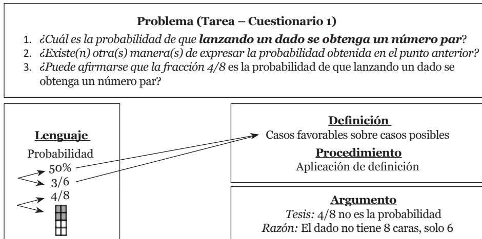
Diagrama 5.12. Configuración final de Jonathan: E_6^{9.4}
