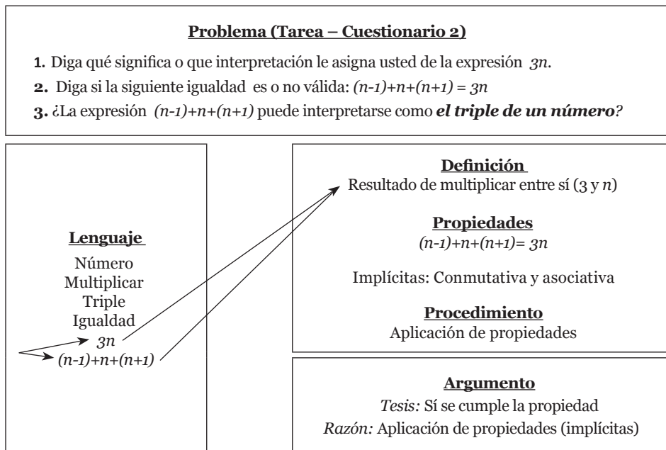
Diagrama 5.14. Configuración inicial de Angely: E_2^{9,1}
