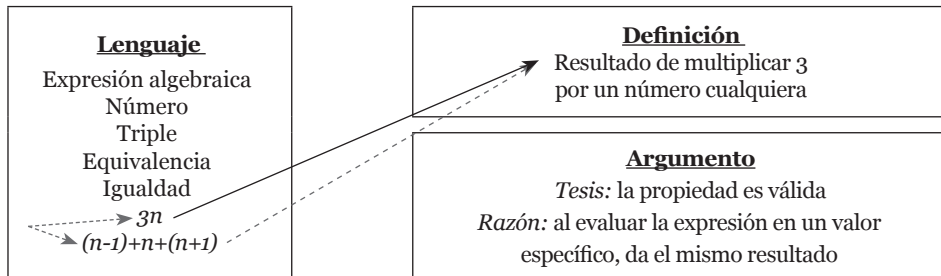
Diagrama 5.16. Configuración final de Cristian: E_1^{9,1}
