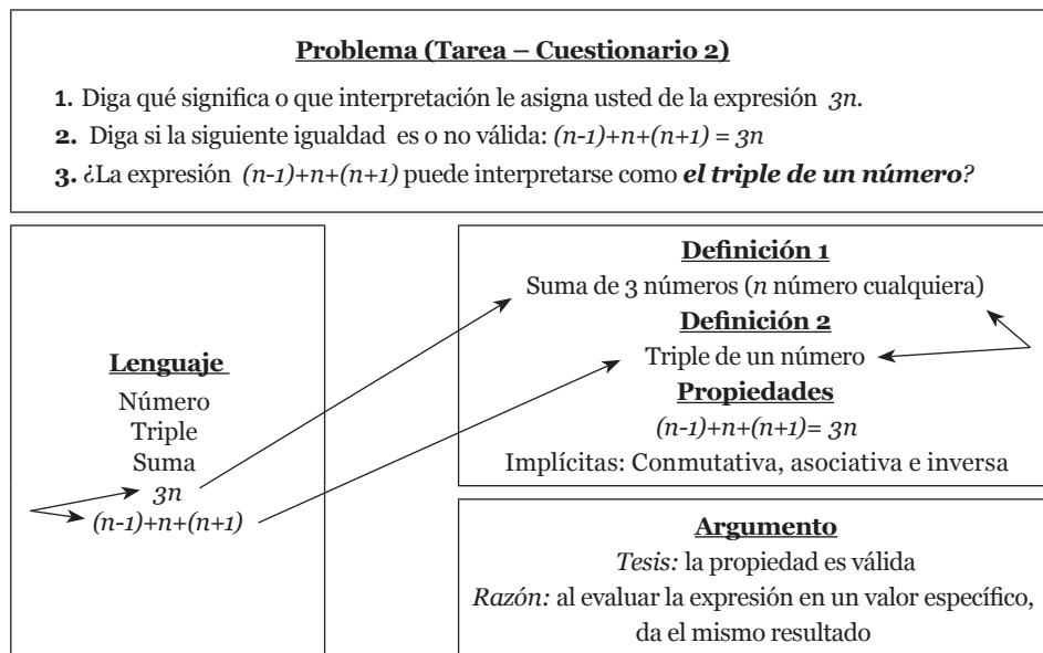
Diagrama 5.18. Configuración final de Dairon: E_3^{9,1}
