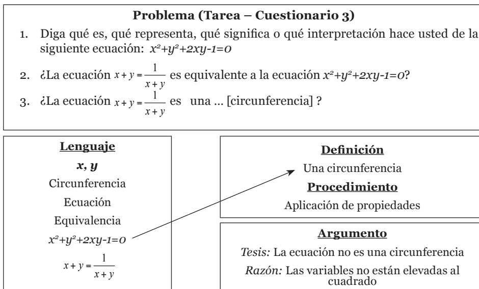
Diagrama 5.2. Configuración inicial de Daniel A.: E 2 11,4
