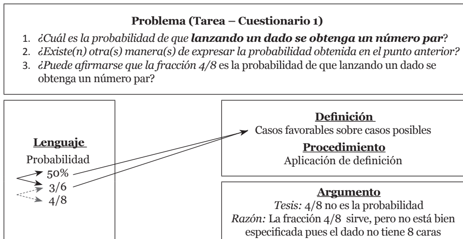
Diagrama 5.10. Configuración final de Pablo: E_4^{9,4}
