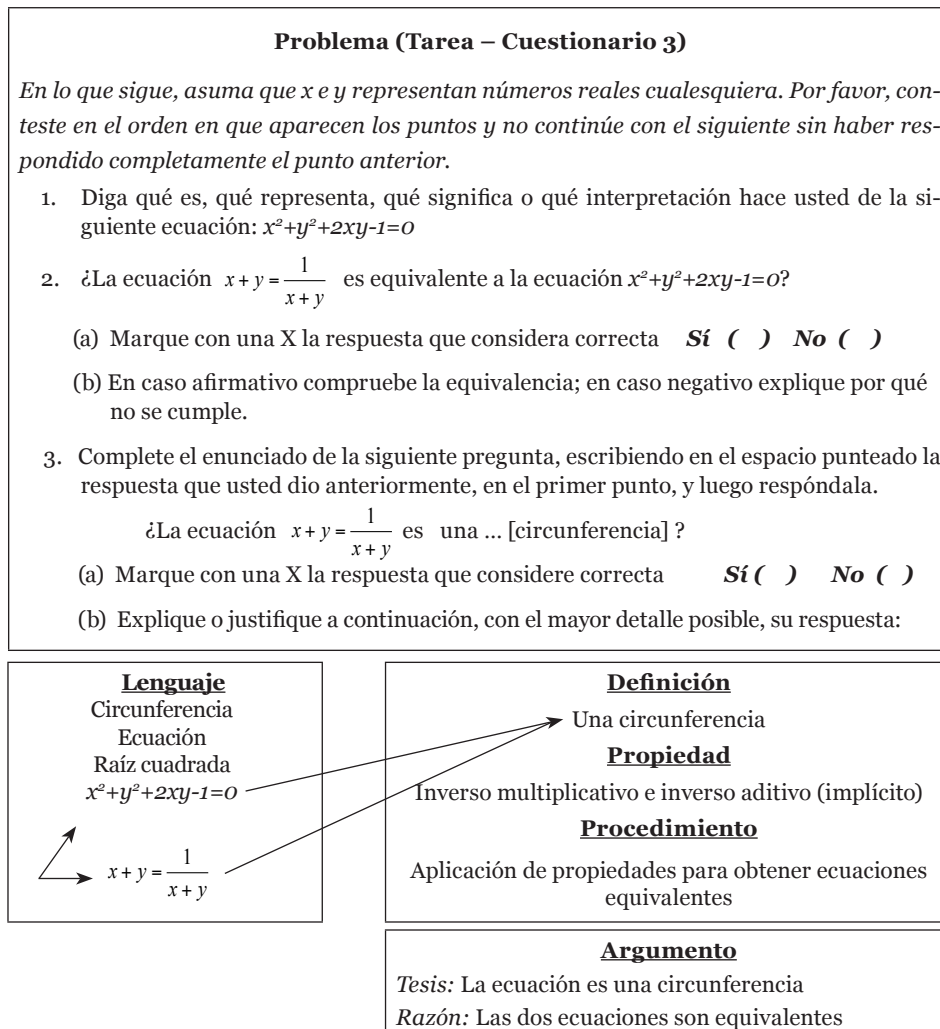
Diagrama 5.1. Configuración inicial de Ma. Elvira: E_1^{11,4}
