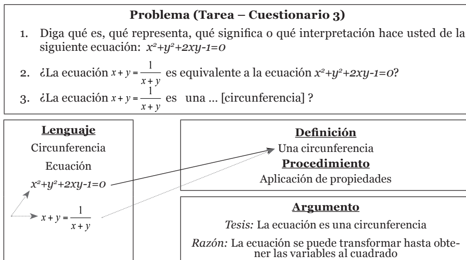
Diagrama 5.5. Configuración final de Daniel A.: E_2^{11,4}
