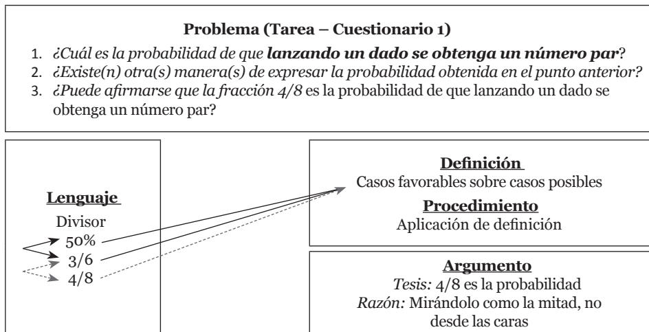
Diagrama 5.11. Configuración final de Daniel: E 5 9,4
