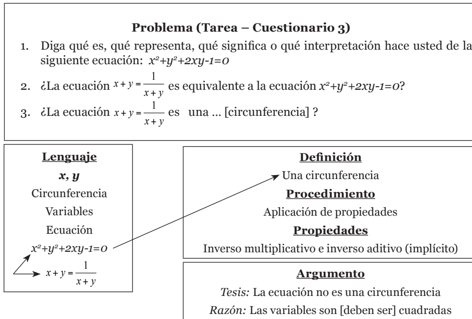
Diagrama 5.3. Configuración inicial de Daniel D.: E_3^{11.4}
