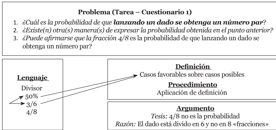
Diagrama 5.8. Configuración inicial de Daniel: E_5^{9,4}
