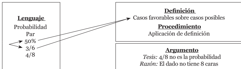
Diagrama 5.7. Configuración inicial de Pablo: E_4^{9.4}
