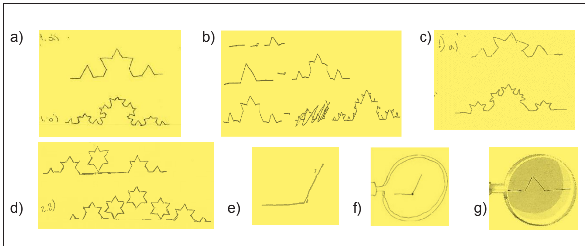
Figura 6. Caso de la CK cerrada
