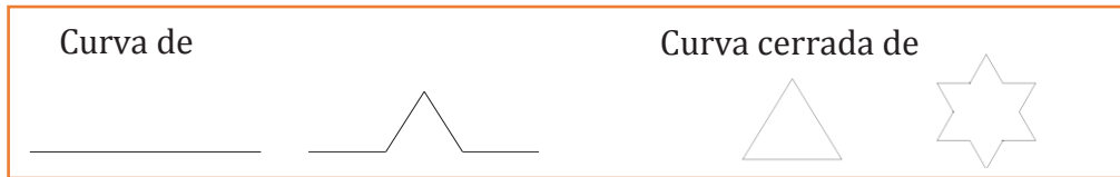
Figura 3. Algoritmo de la construcción geométrica para curva abierta y curva cerrada de Koch
