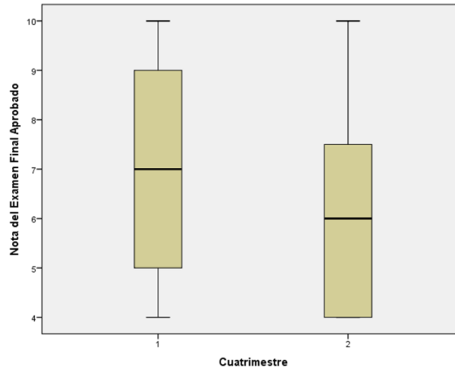
Gráfico 3. Box-Plot- Calificaciones de los Exámenes Finales por Cuatrimestre
