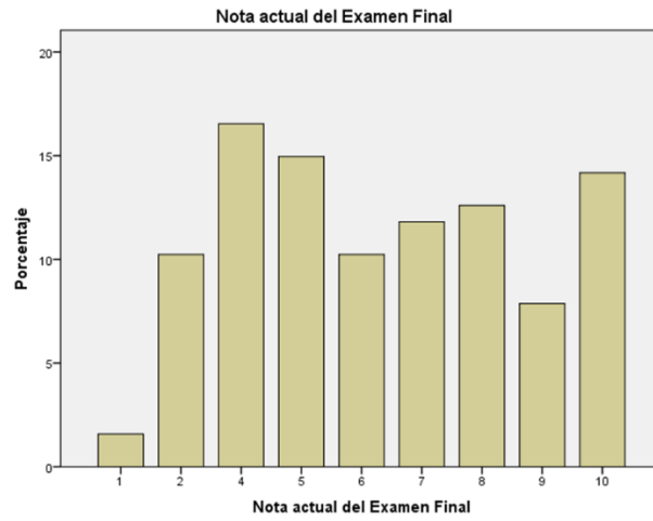
Gráfico 4. Calificaciones obtenidas en los Exámenes Finales
