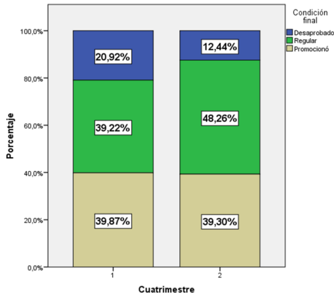
Gráfico 1. Condición Final de Cursada por Cuatrimestre
