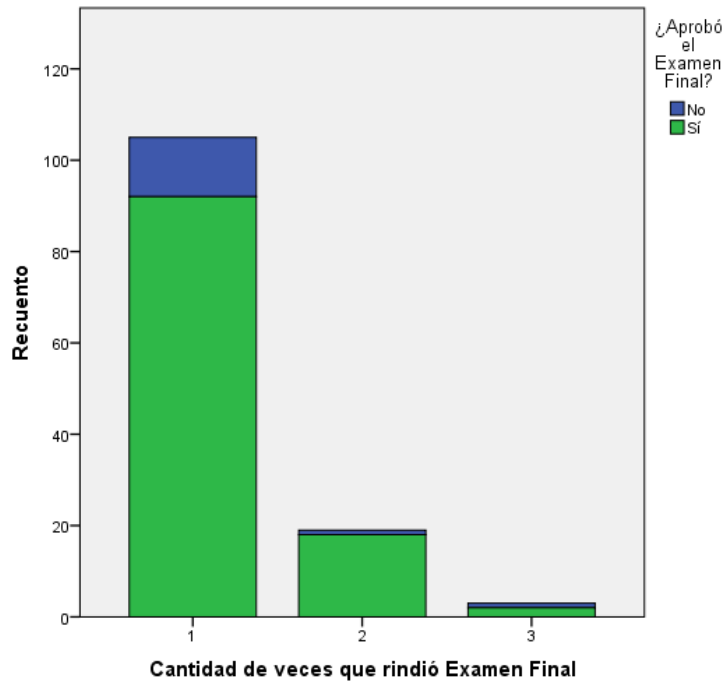
Gráfico 5. Cantidad de veces que rindió Examen Final
