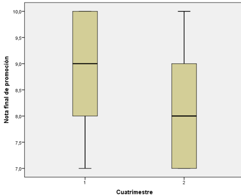
Gráfico 2. Box-Plot-Calificaciones de los Exámenes Promocionales por Cuatrimestre
