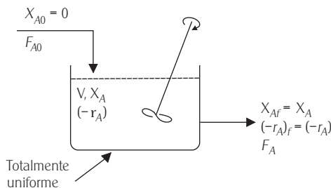
Figura 1 Reactor químico
