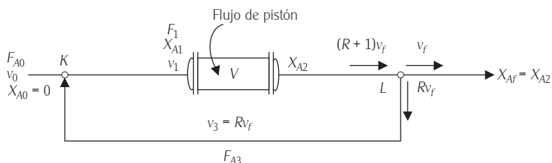
Figura 6 Nomenclatura empleada en un reactor con recirculación
