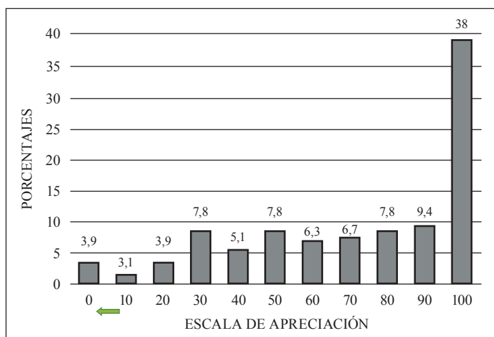
Figura 3. Porcentaje de respuestas al ítem 5 según escala de apreciación (respuesta esperada bajo 10), n = 257
