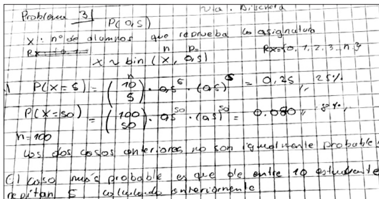
Figura 6. Argumentación correcta según modelo binomial del estudiante 02
