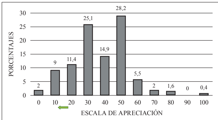
Figura 4. Porcentaje de respuestas al ítem 7 según escala de apreciación (respuesta esperada bajo 20), n = 257
