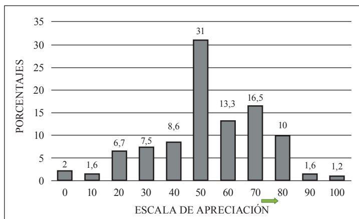
Figura 2. Porcentaje de respuestas al ítem 3 según escala de apreciación (respuesta esperada sobre 75), n = 257
