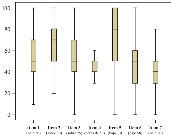
Figura 1. Distribución de respuestas a 7 ítems (respuesta esperada) según escala de apreciación, n = 257
