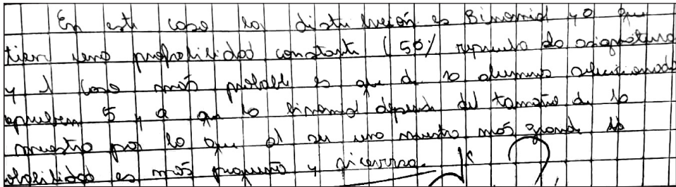
Figura 5. Argumentación correcta según tamaño muestral del estudiante 01
