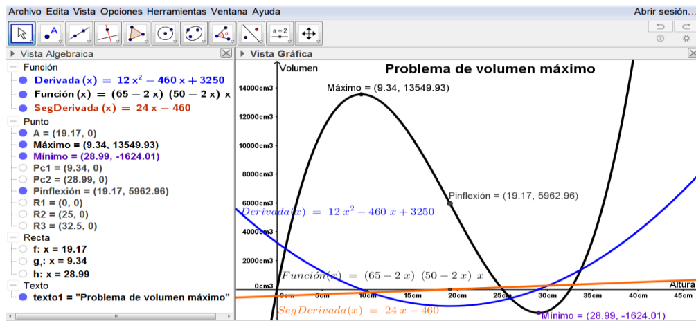
Figura 6. Análisis de la función de volumen máximo con Geogebra.
