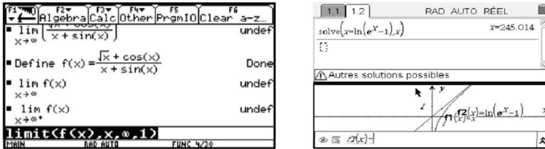
Figura 7. Resultados falsos entregados por una calculadora simbólica
