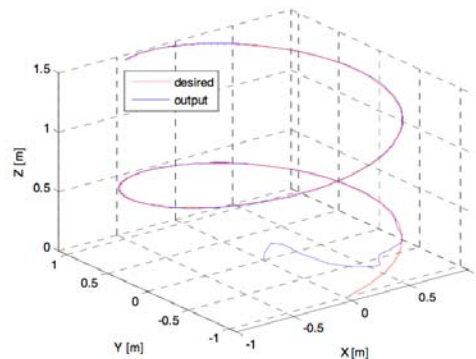
Figura 3. Evolución de la posición del cuadrirotor.
