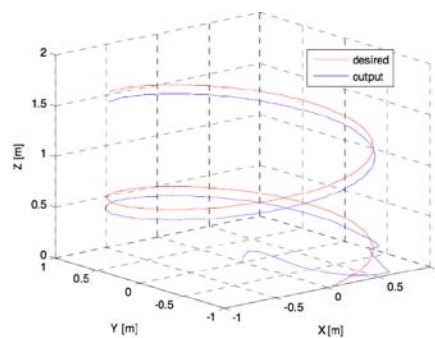
Figura 4. Evolución de la posición del cuadrirotor, con un error de los parámetros del 20%.
