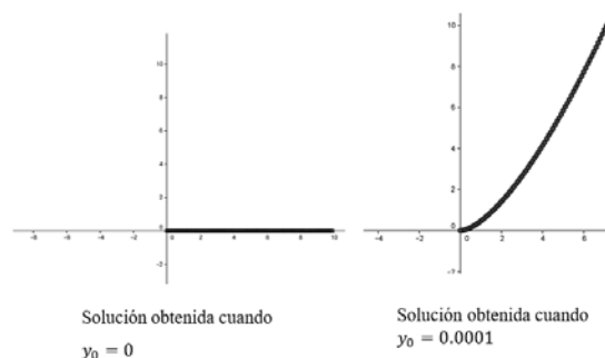
Figura 1. Aproximaciones numéricas de la solución de la ecuación diferencial alrededor de (0,0) que da el método de las quebradas
