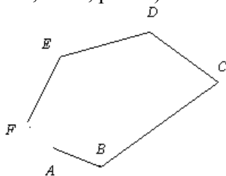
Figura 7. Al dibujar el espacio real identificado por polígono cerrado ABCDEA , con transportador y regla graduada, a cierta escala, este no cierra debido a los errores de observación de las distancias cometidos con el grafómetro y cordel, quedando así el polígono abierto ABCDEF .
