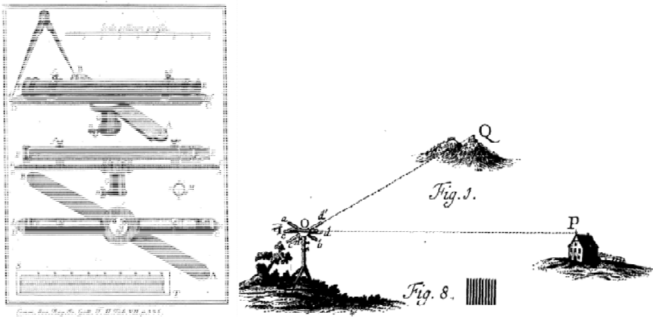
Figura 4. A la izquierda, grafómetro alemán con anteojo, la abertura del compás servía para determinar el valor angular apreciando su valor sobre la escala que ahí aparece. A la derecha se puede ver el método utilizado en la medición de un ángulo horizontal. Fue utilizado para los levantamientos topográficos alrededor del año de 1750.
