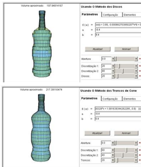
Cálculo do volume utilizando aproximação com o Método dos Troncos
