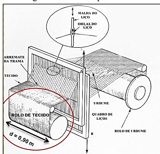
Figura 4 – Os componentes de um tear
