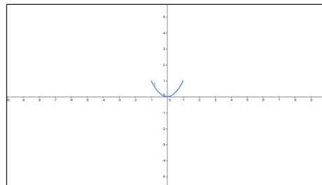
Figura 4. Función[x^2, -1, 1]
