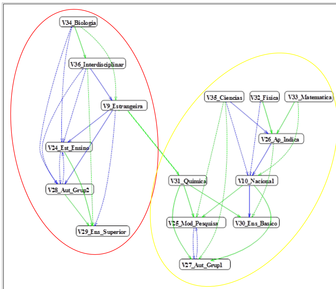
Figura 2. Gráfico implicativo com os fechamentos transitivos.
