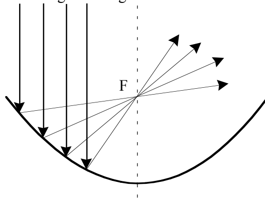
Figura 25. Propiedad óptica de la parábola y principio de la física
